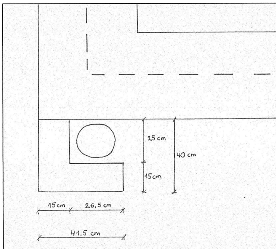
Rys. 1 Szkic obudowania rur spustowych
